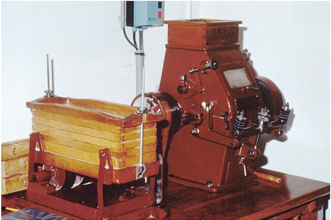
Atelier de fabrication (L), 1er étage : appareil à cylindres et plansichter du laboratoire.
