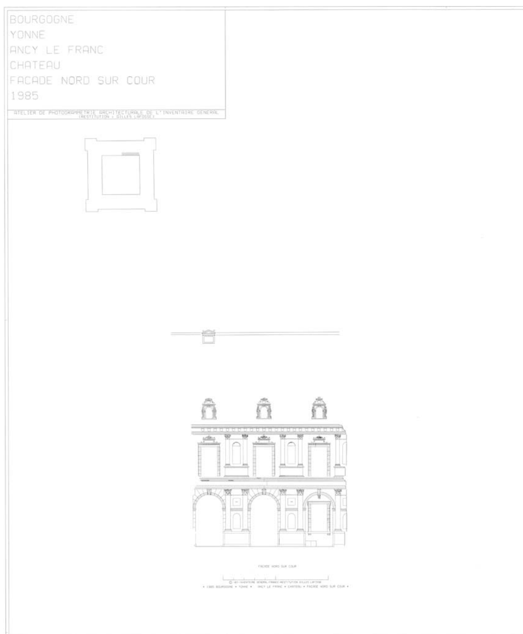
Façade nord sur cour, restitution photogrammétrique.
