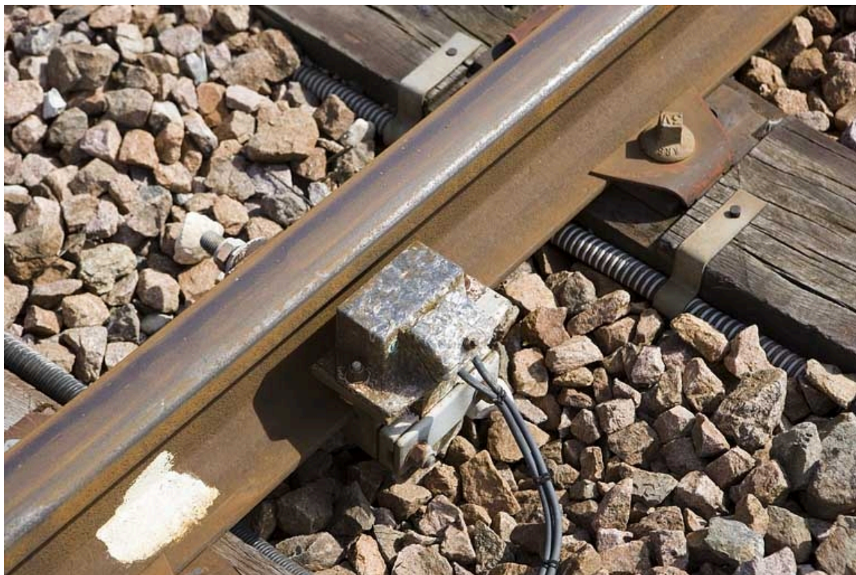
Pédale électronique.
