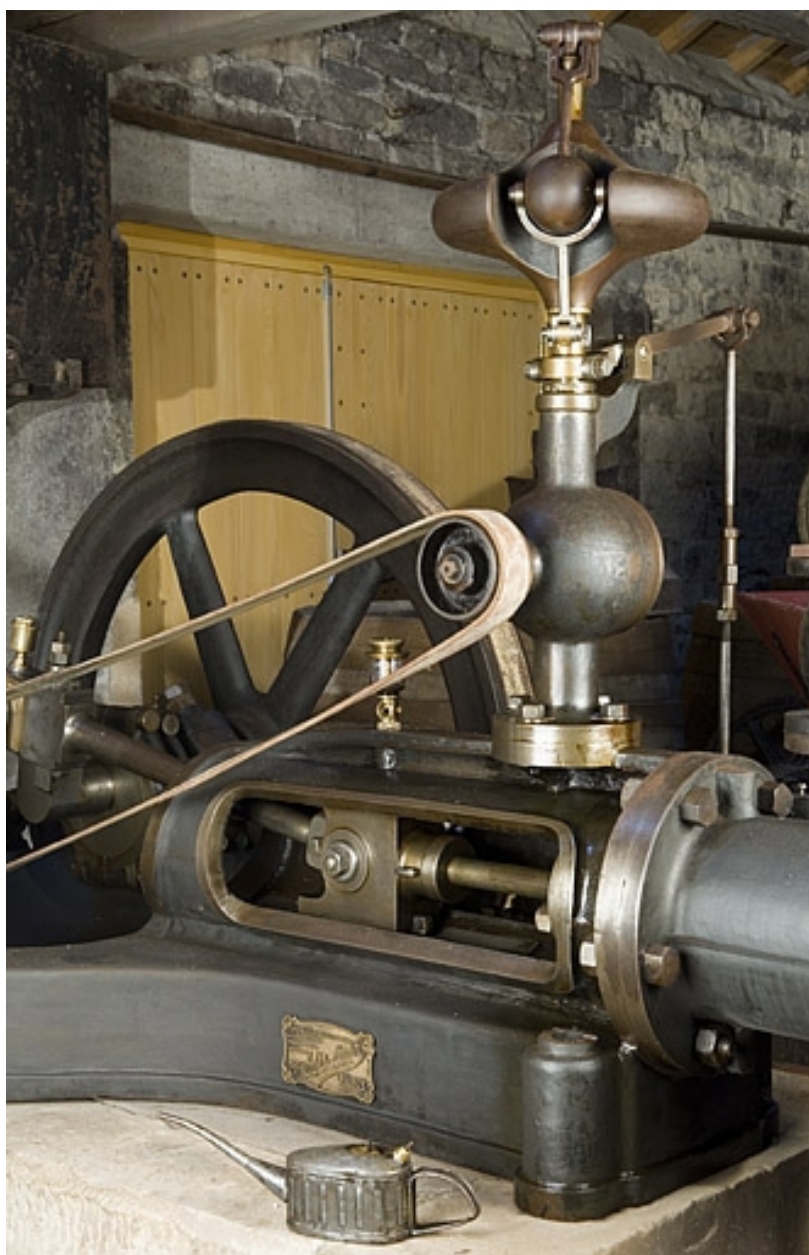
Machine à vapeur Diebold et Michel (Nancy). Détail.
