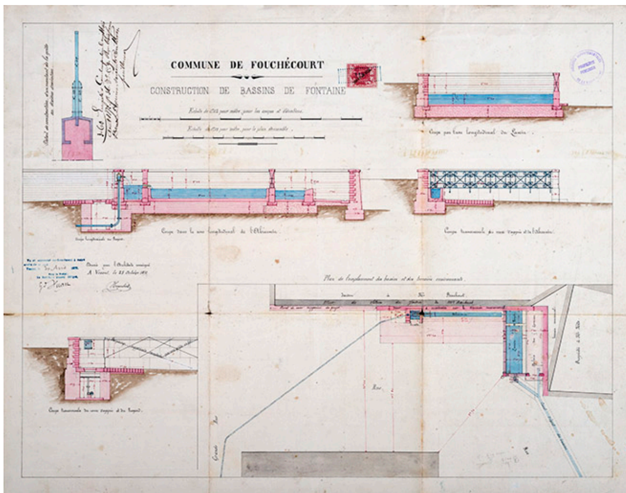
Projet de construction de bassins (1871).
