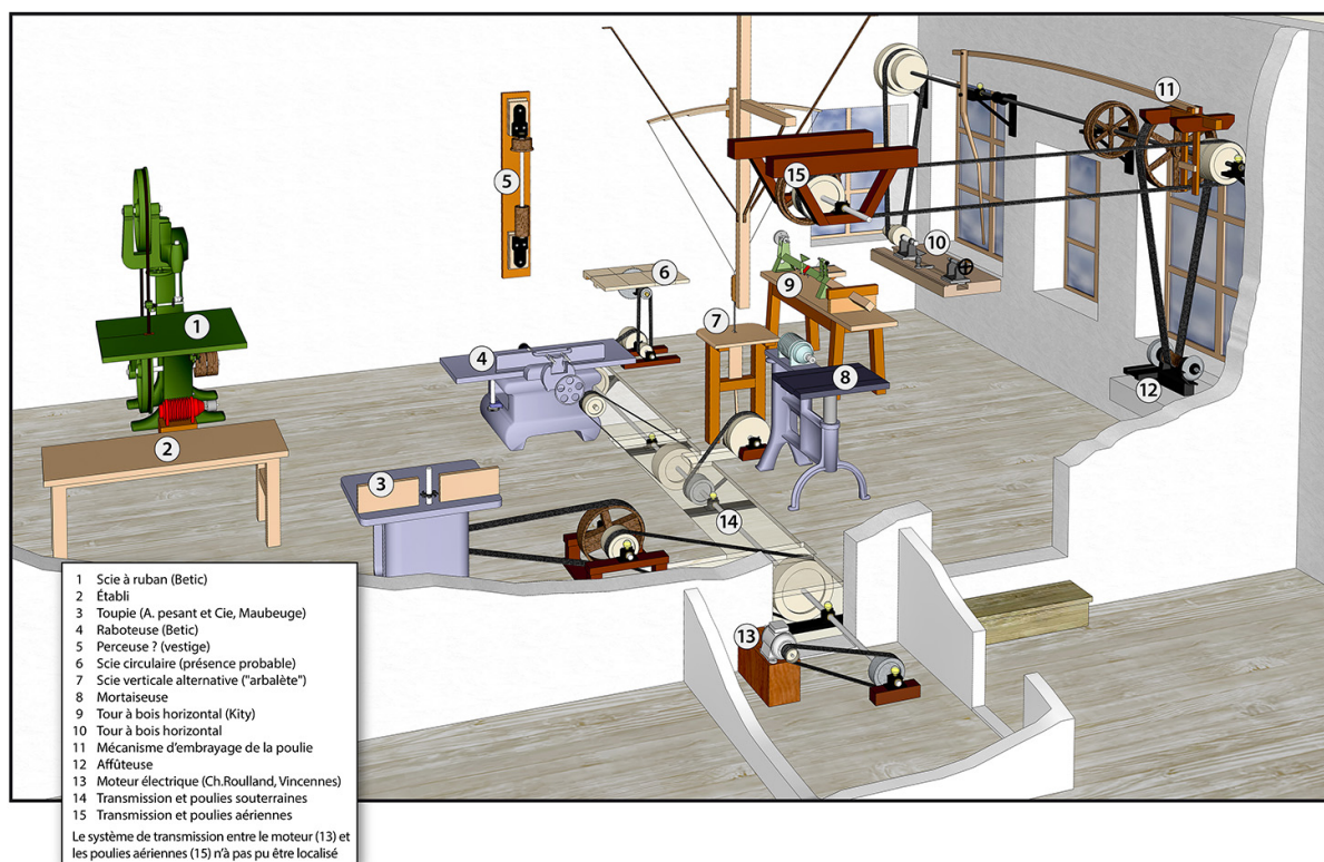
Menuiserie Baudiquey (Sancey-le-Long). Plan de disposition des machines à l'étage de soubassement
