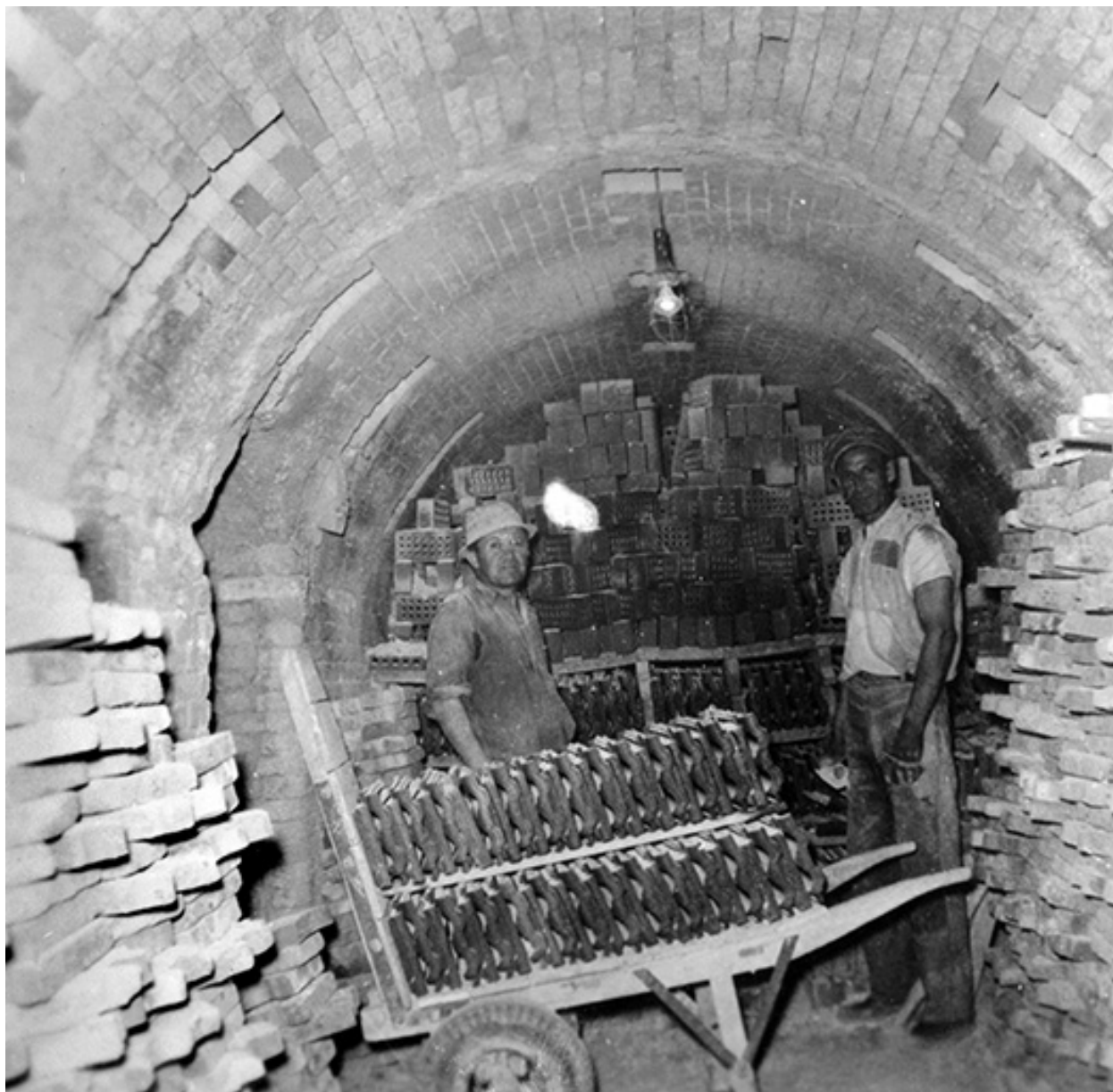
Briqueterie et tuilerie Emile Jacob, Commenailles : déchargement du four Hoffmann, 1955.
