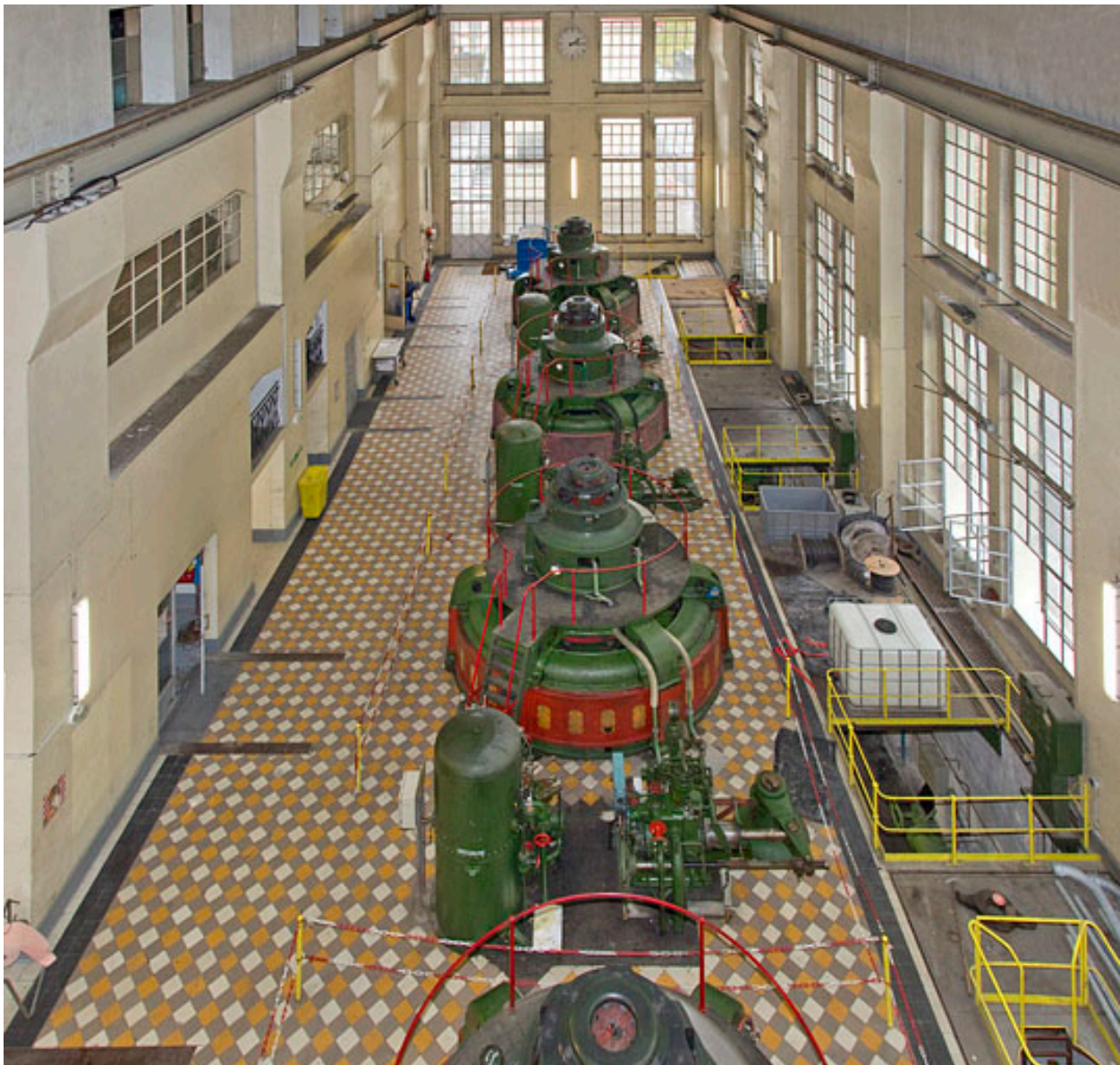
Centrale hydroélectrique de Liebvillers : intérieur.
