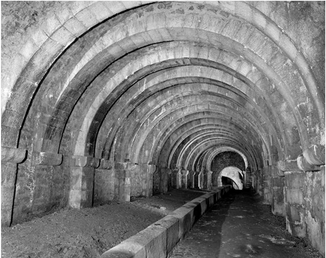
Galerie de communication entre les puis d'Amont et d'Aval (1993).
