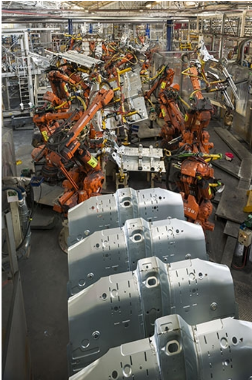
Atelier de ferrage. Soudage des pièces de la caisse en blanc dans un îlot robotisé (4).
