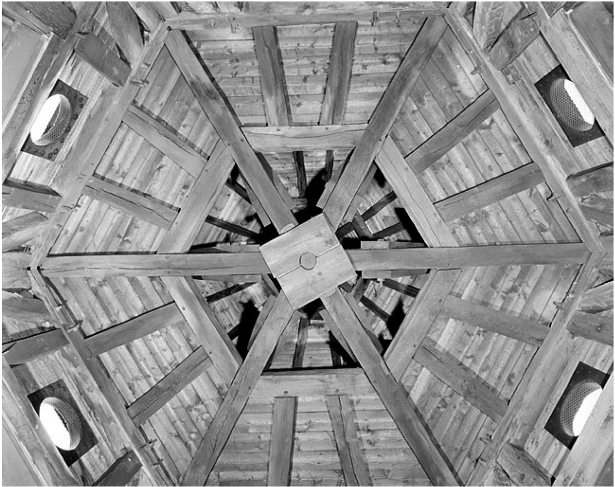
Tour Henriette. Charpente du lanteron.
