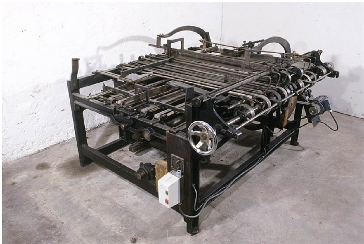
Machine à plier (plieuse Mentges Folder Co. de l'ensemble de la presse à cylindre Voirin) : vue d'ensemble
