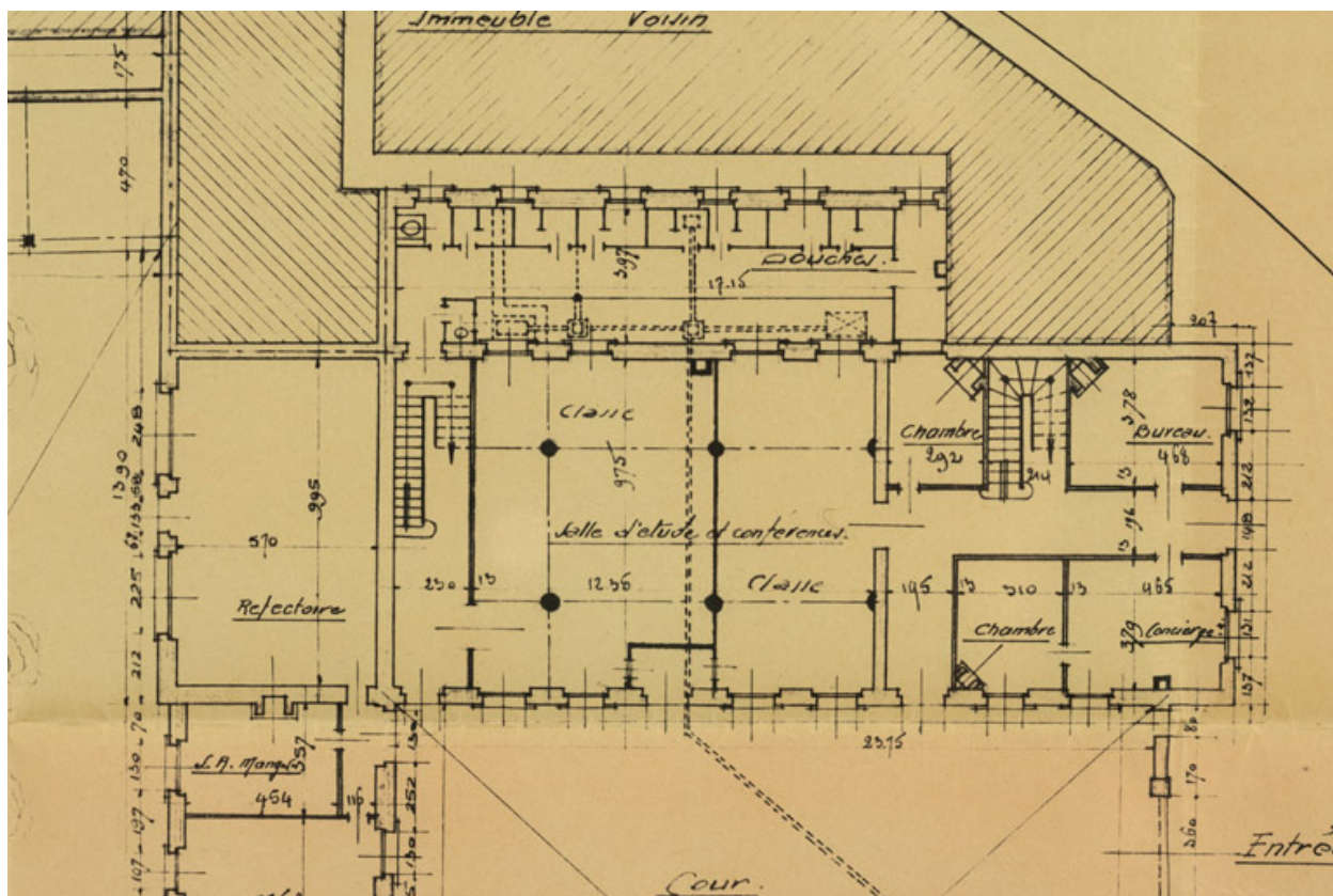
Collège de Cosne-s-Loire [état actuel]. Plan d'ensemble du rez de chaussée [détail de l'ancienne église]. 1936.
