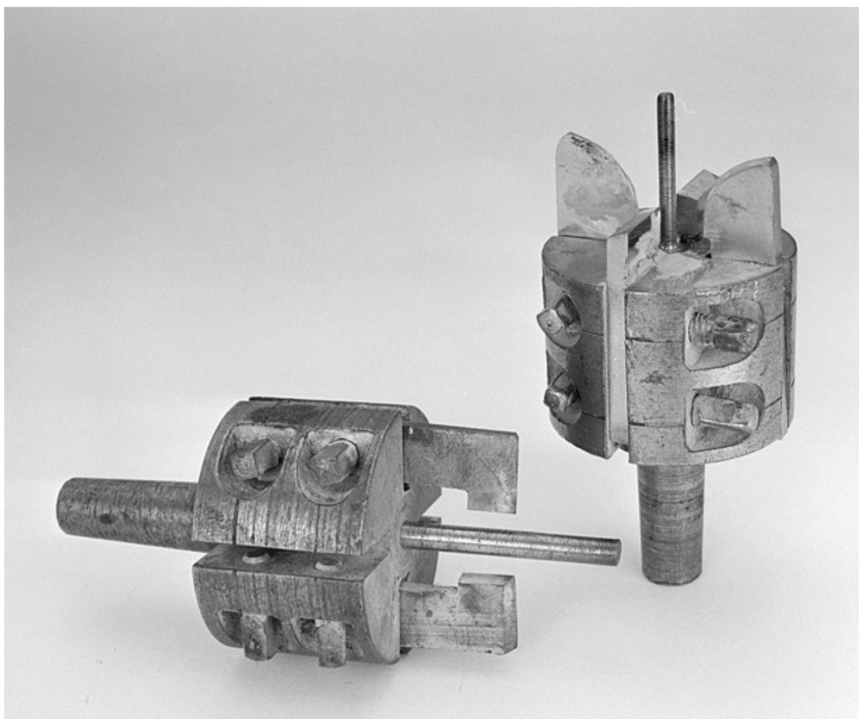
Détail de deux outils de coupe.
