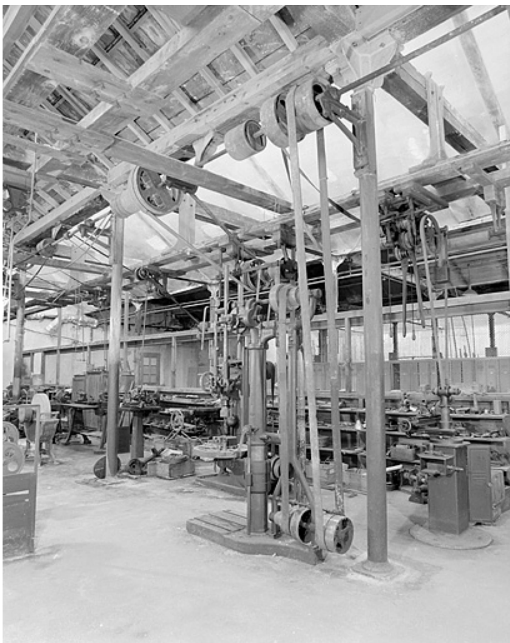
Atelier de mécanique. Transmission par courroies verticales de la perceuse à colonne.
