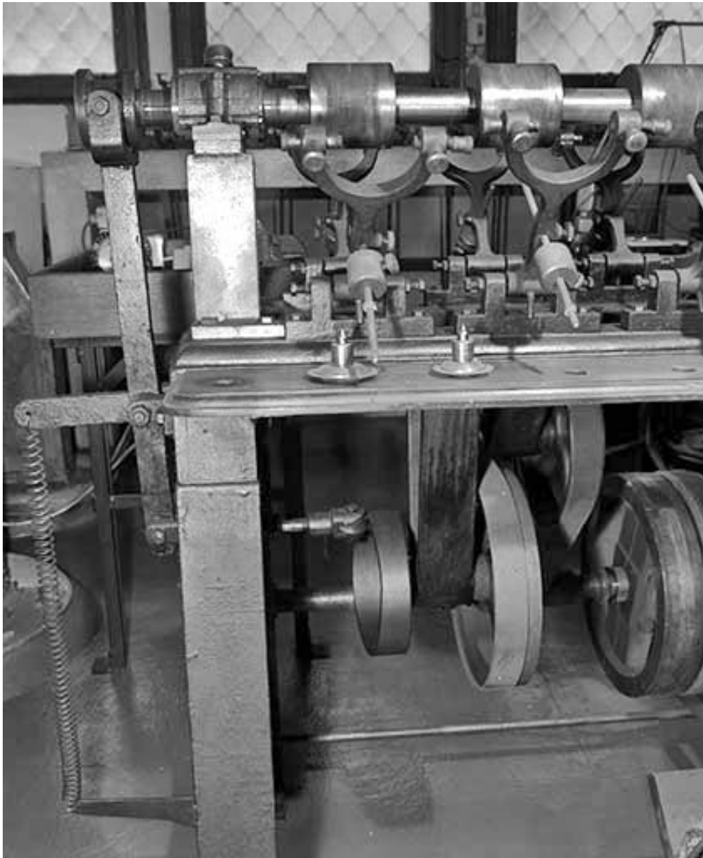
Détail montrant deux emplacements de diamantage.
