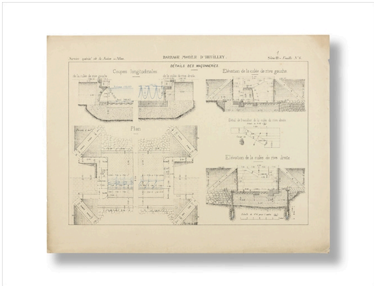
Barrage mobile d'Heuilley. Détail des maçonneries. 1886.
