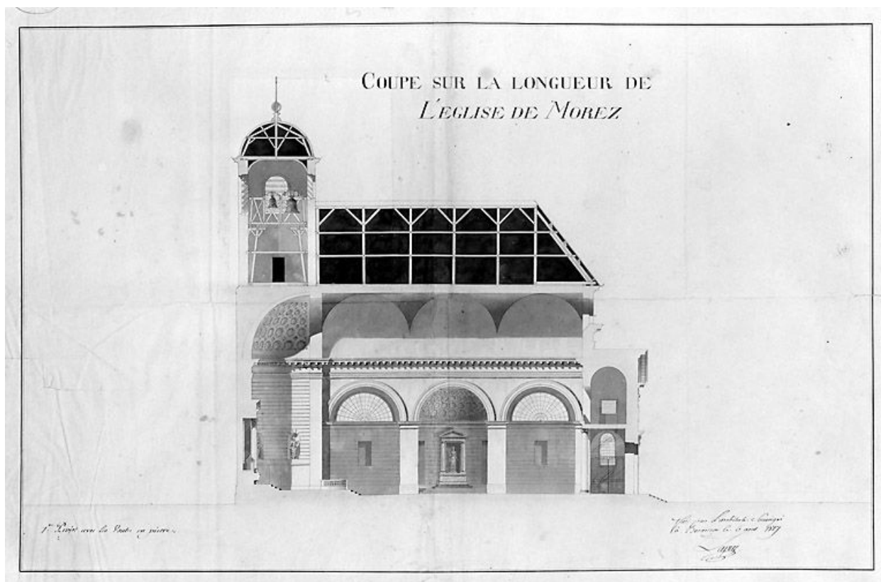
Coupe sur la longueur de l'église de Morez, 1817. Dessin (plume, lavis), 6 août 1817, échelle approximative 1:120. Porte en note : 1er projet avec les voûtes en pierre.
