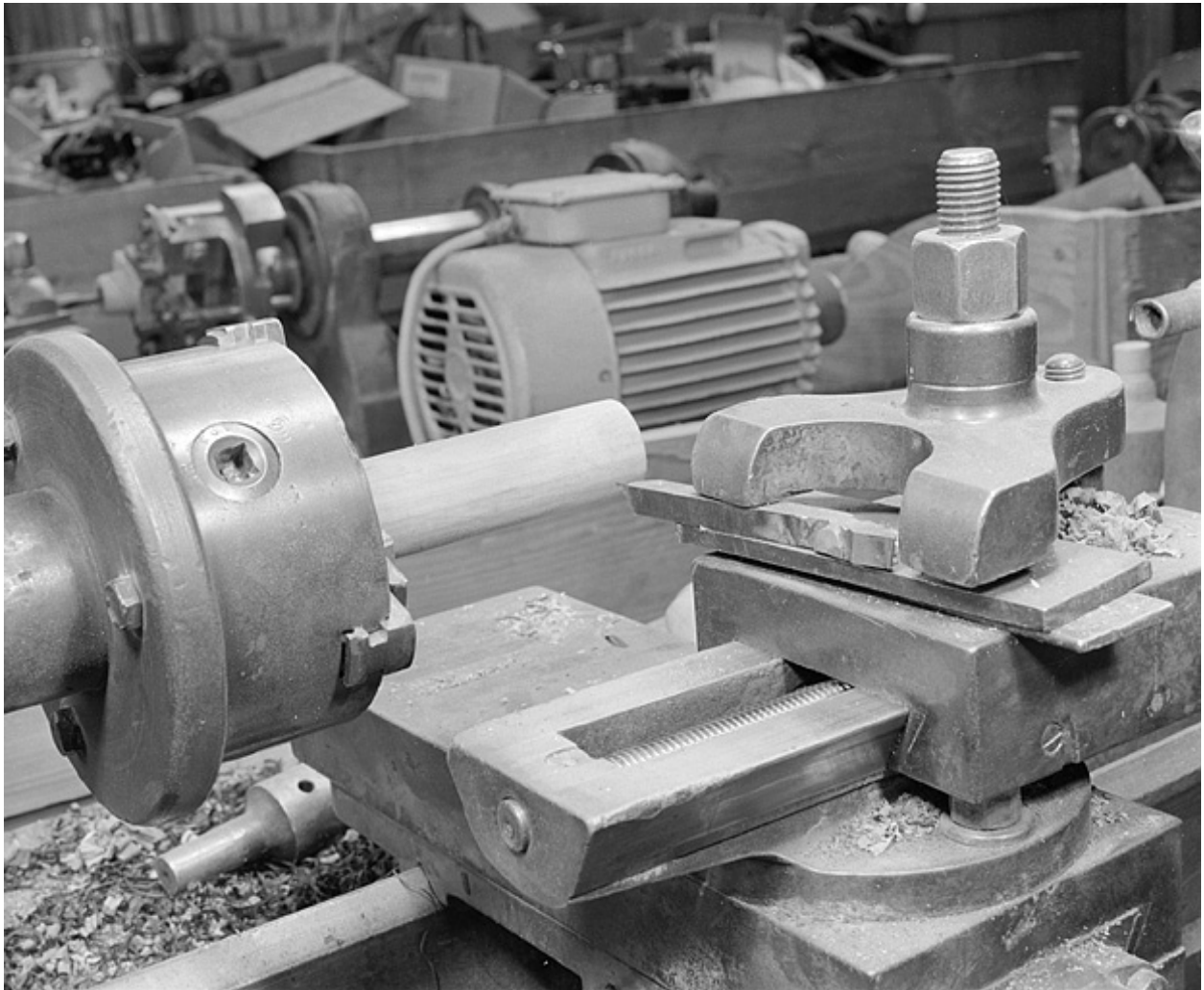
La poupée fixe et le traînard, vus de trois quarts gauche.
