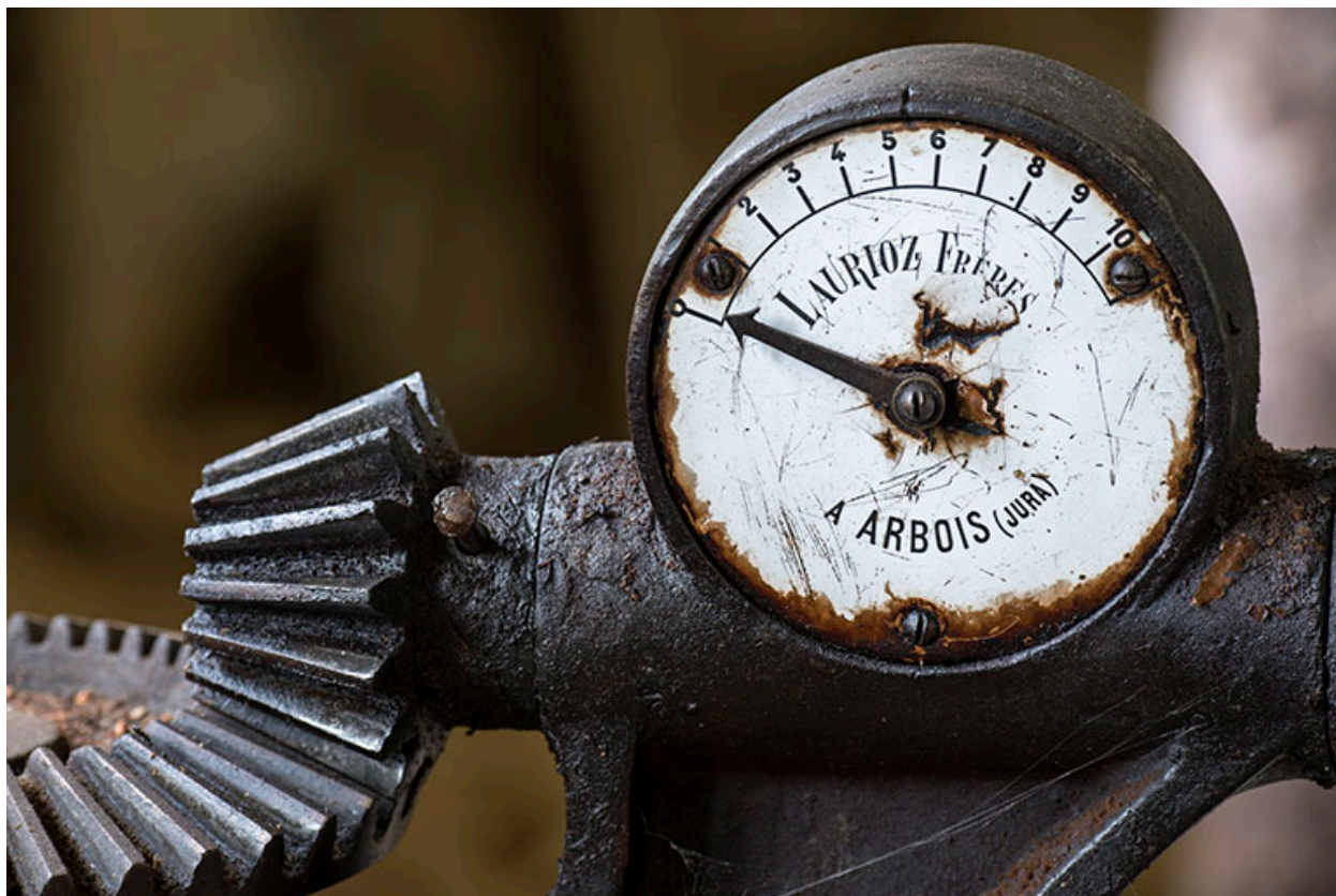
Manomètre de turbine Laurioz (usine d'outillage Louis Garnache-Chiquet et Fils, Les Gras).
