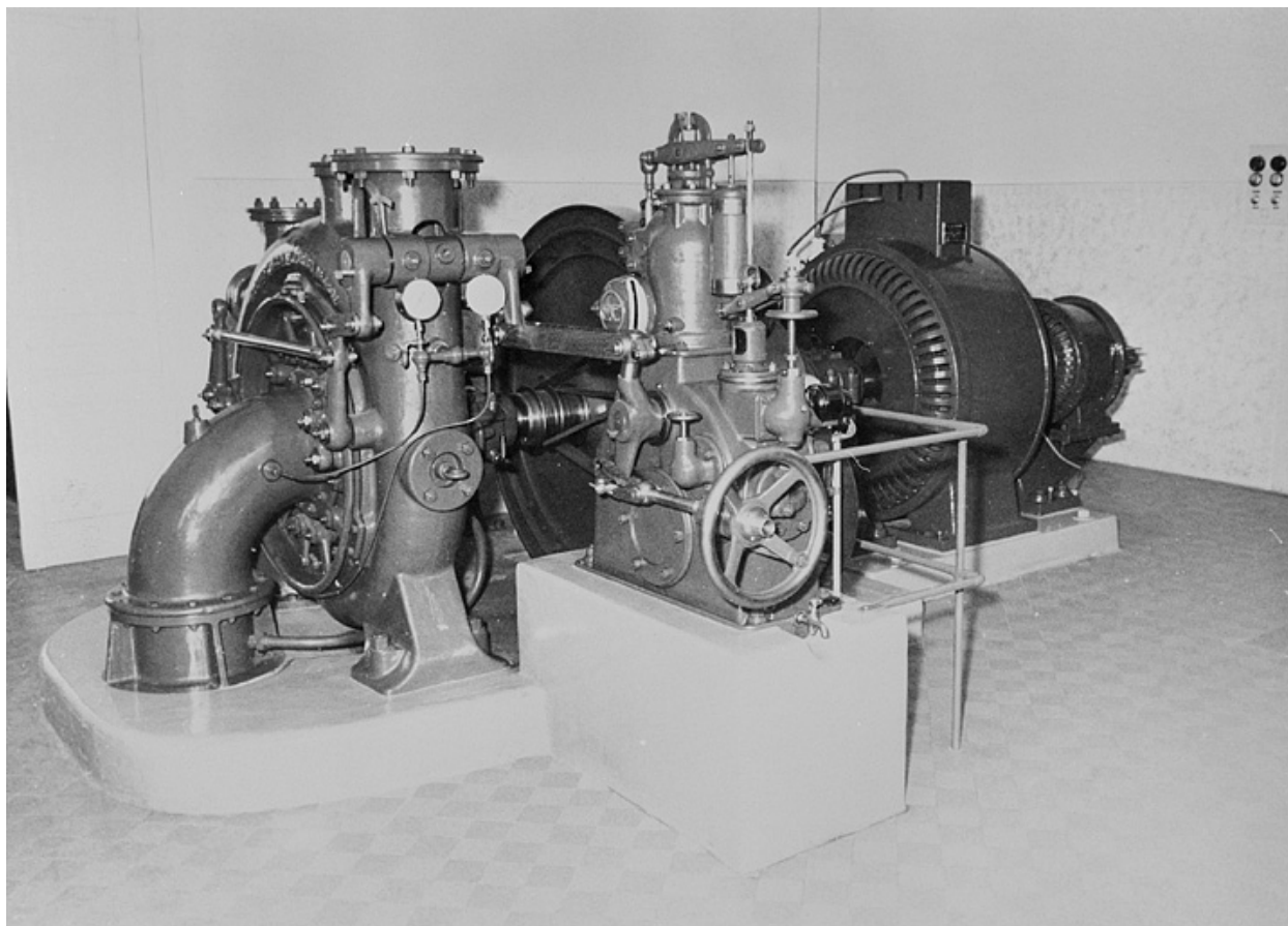
Usine du Flumen. Groupe Escher-Wyss Bréguet de 1911.
